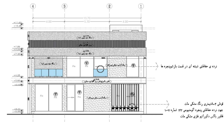
نمای شرقی EAST
